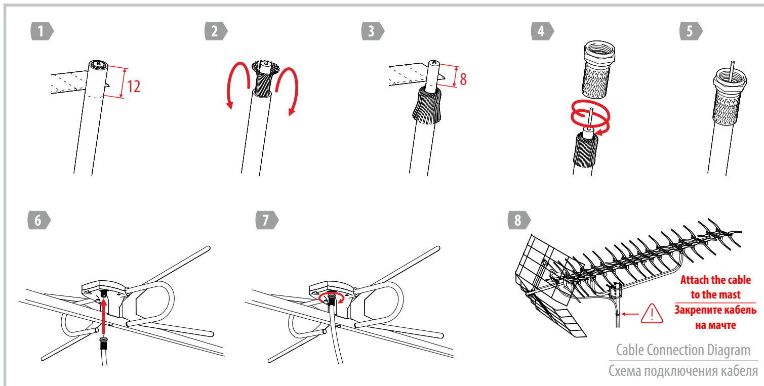
Mount Assembly Diagram Схема сборки узла крепления
