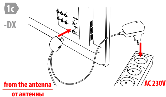
Cable Connection Diagram Схема подключения кабеля
