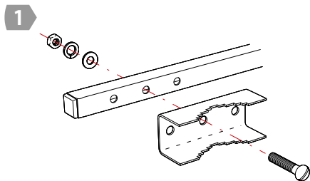
Reflector Assembly Diagram Схема сборки рефлектора
