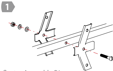
Reflector Assembly Diagram Схема сборки рефлектора
